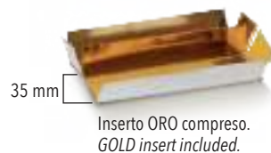
QUADRETTO + fascetta + inserto 35 mm 145x75x35 | 133631S 145x145x35 | 133632S 215x145x35 | 133633S Vedi a pagina 61. See page 61.
